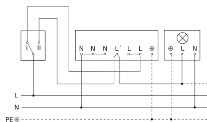
Diagrama electrónico conexión del acoplador pulsador de 4 vías al APC DALI2
