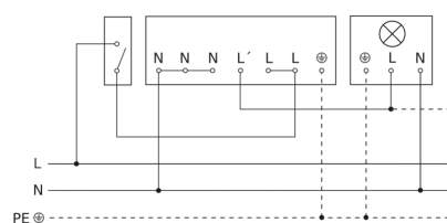
Diagrama electrónico lámpara con conductor neutro
